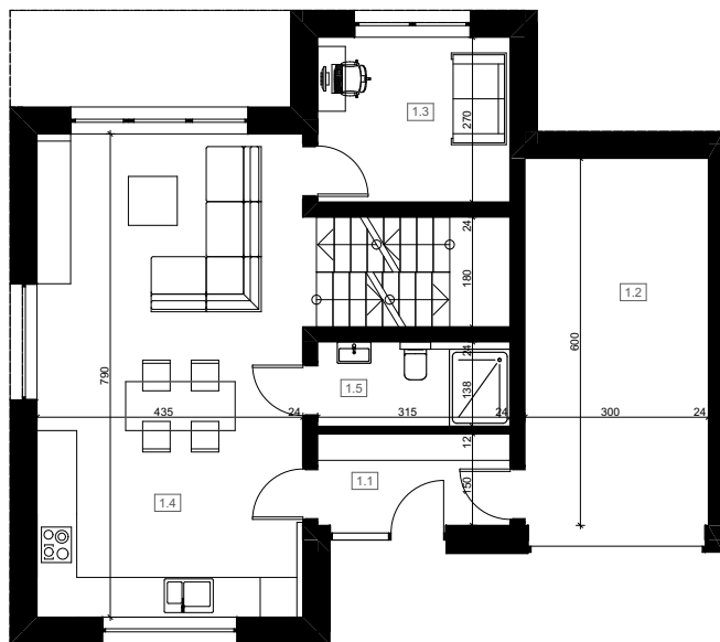
RZUT PARTERU
