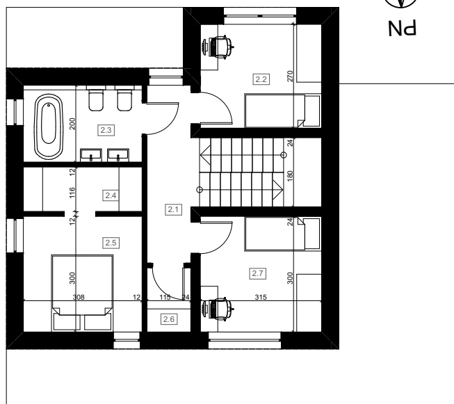
RZUT PIĘTRA
