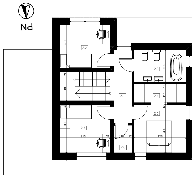
RZUT PIĘTRA
